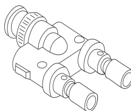
图二 BNC 公头转双接线柱
