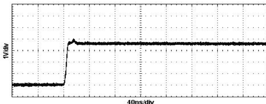
未添加延长线的波形
