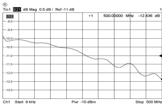
图 1 频响曲线
