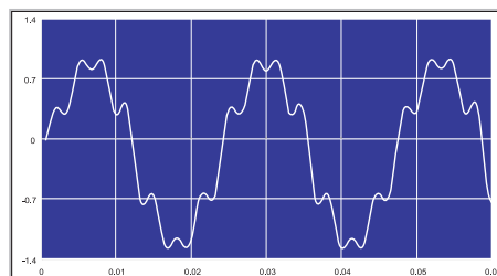
谐波波形
