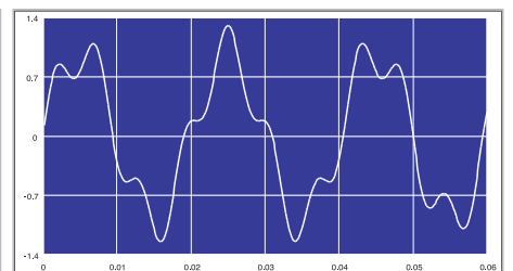
间谐波波形
